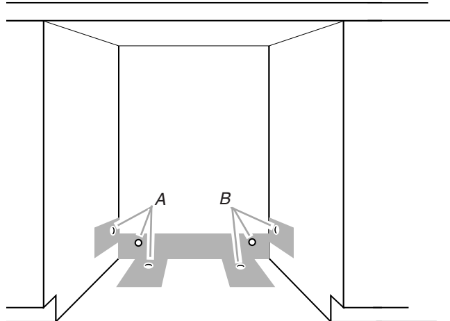
A. Ubicaciones opcionales del orificio para el alambre directo B. Ubicaciones recomendadas para el orificio
