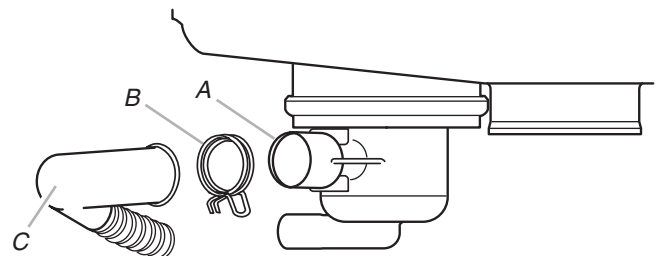
A. Conector de desagüe B. Abrazadera tipo resorte para manguera de desagüe C. Manguera de desagüe
