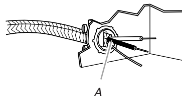
A. Alambre directo
