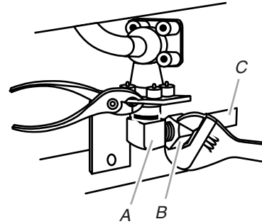
A. Codo en la válvula de entrada de agua B. Tuerca de conexión de compresión C. Tubo de cobre
