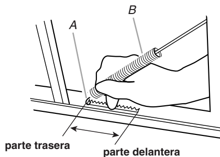
A. Extremo del resorte B. Resorte
